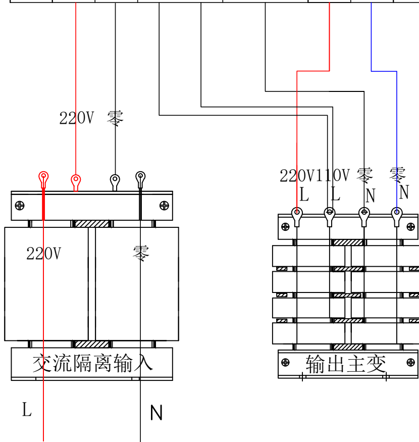
电网市电输入
